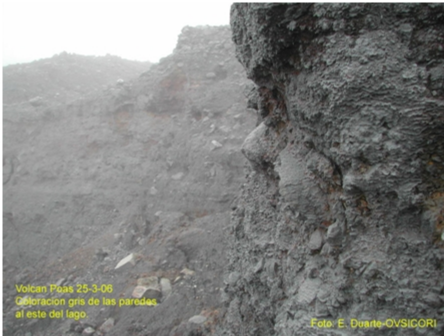
Figura 19: Pared Este del cráter cubierta con sedimentos finos del fondo de la Laguna Caliente, emitidos por una erupción freática que ocurrió la noche del 24 de marzo, 200t.
