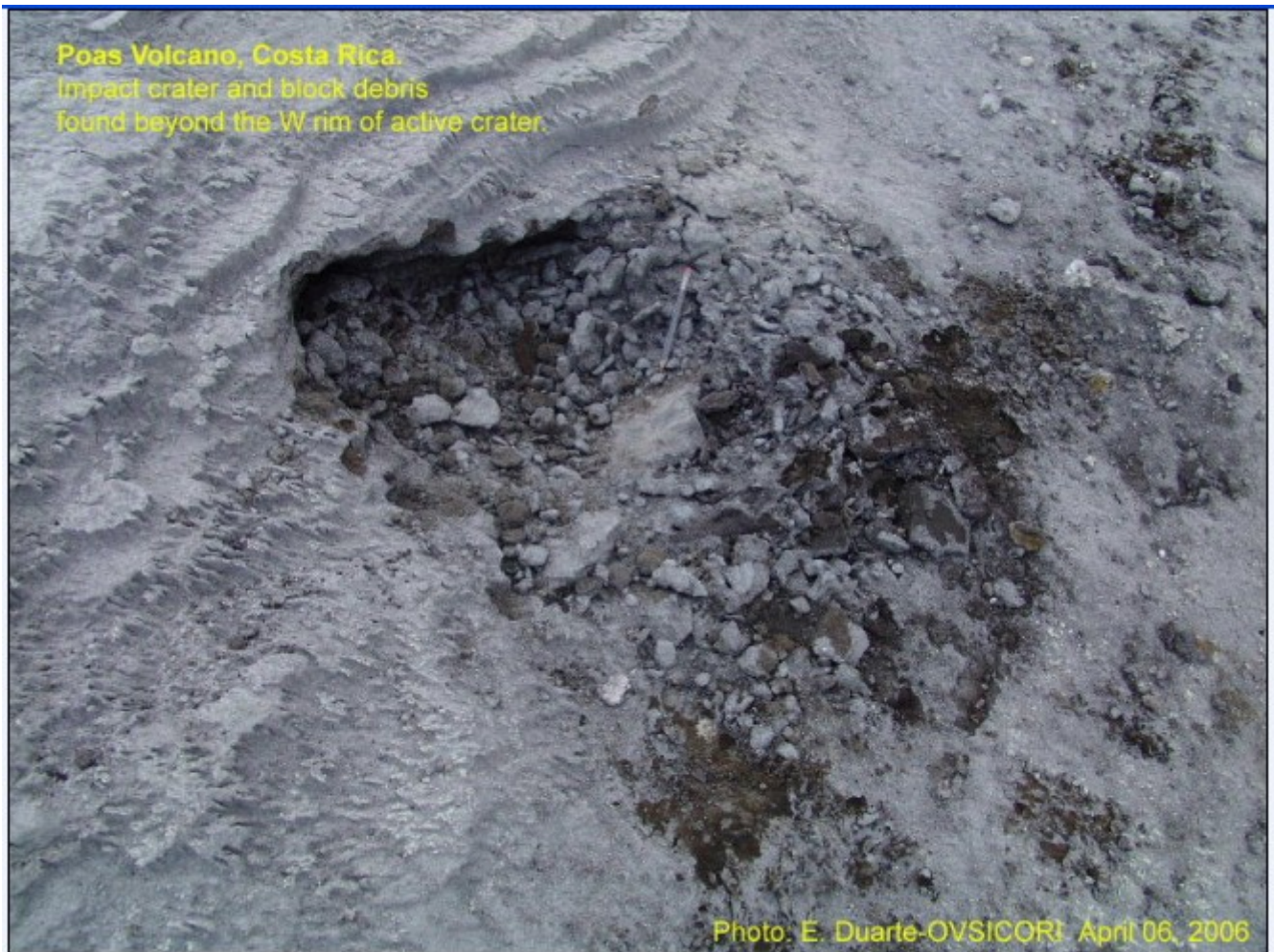
Figura 30: Cráteres de impacto observados al oeste de Laguna Caliente, probablemente producidos durante la erupción de marzo 26 por la noche.
