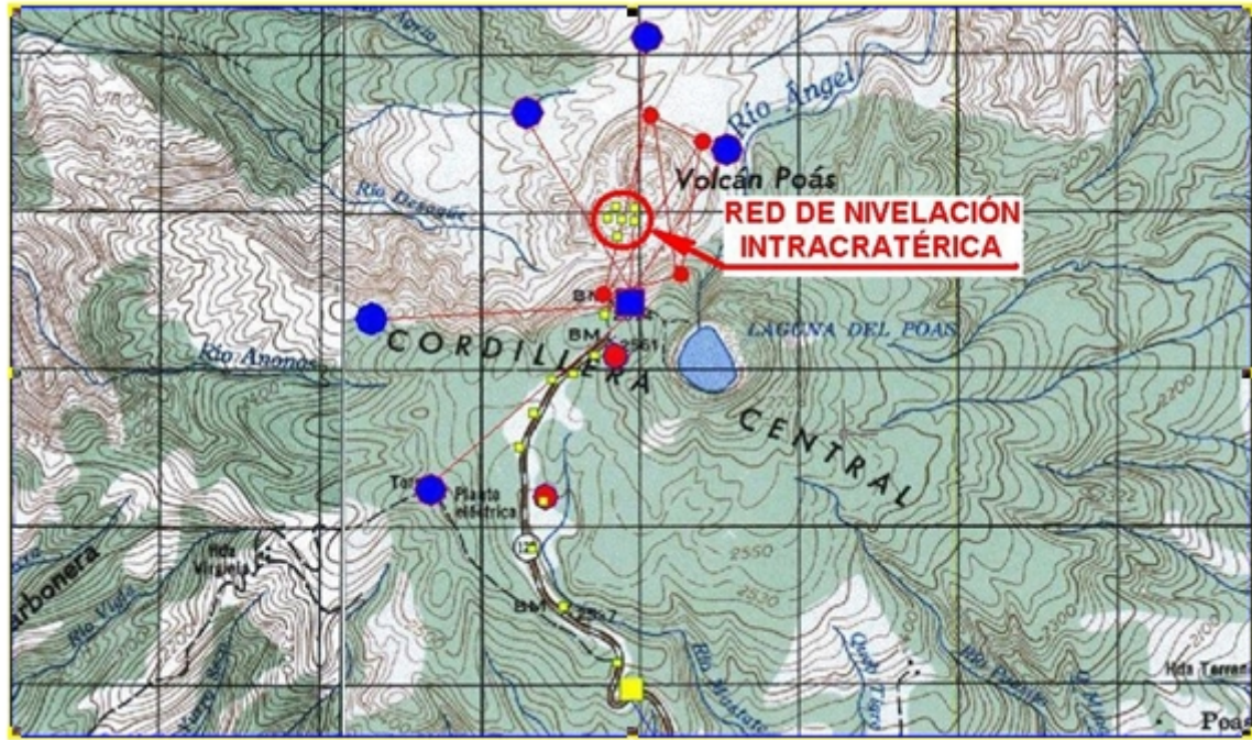
Figura 13: Red de deformación del volcán Poás. El cuadrado azul indica la ubicación del pilar y los círculos azules indican la ubicación de los reflectores fijos.
