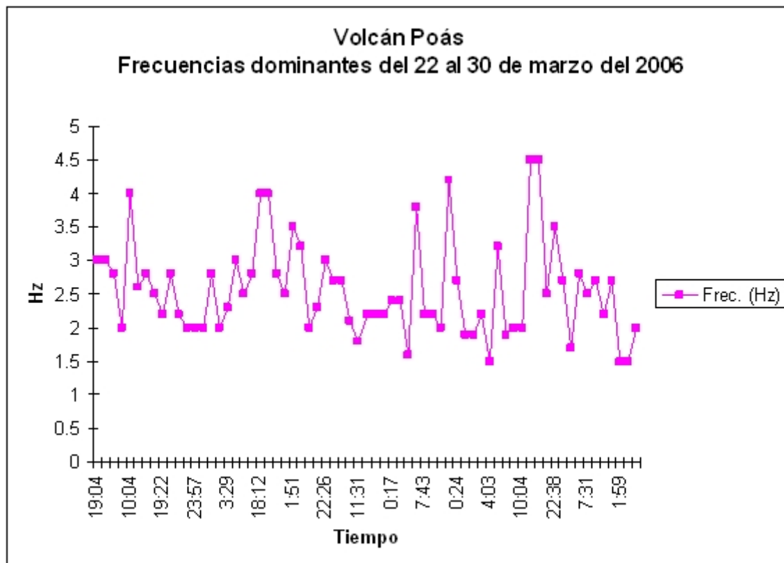
Figura 9: Frecuencia de los sismos de frecuencia intermedia (AB) que siguieron a la señal de ruptura de sellos ocurrida el 21 de marzo, 2006. El eje horizontal es tiempo en horas.
