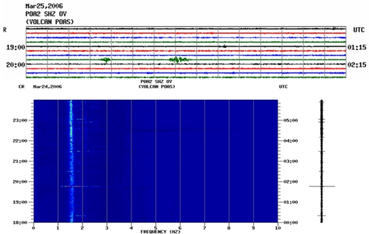
Figura 11: Espectrograma de la erupción freática ocurrida el 24 de marzo a las 19:51 hrs hora local (01:51 hrs GMT). La frecuencia dominante (1.5 Hz) corresponde al tremor monocromático armónico. Note que esta erupción freática fue precedida por una erupción freática más pequeña a las 01:48 hrs GMT.
