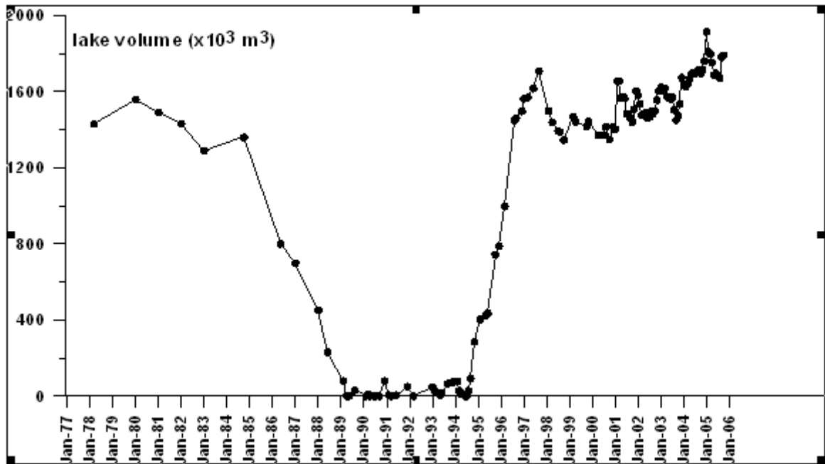
Figura 6: Variación en el volumen de la Laguna Caliente, lago del cráter principal del Poás, 1977-2006. La profundidad del lago era de unos 45 m al final de 2005. Note que el lago incrementó su temperatura de 51 °C el 28 de febrero de 2006 a 54 °C el 01 de abril de 2006, pero en contraste, el pH del lago alcanzó un mínimo de 0.59 el 28 de febrero de 2006. Este pH se incrementó a 0.65 para el 01 de abril y a 0.71 para el 06 de abril, 2006.
