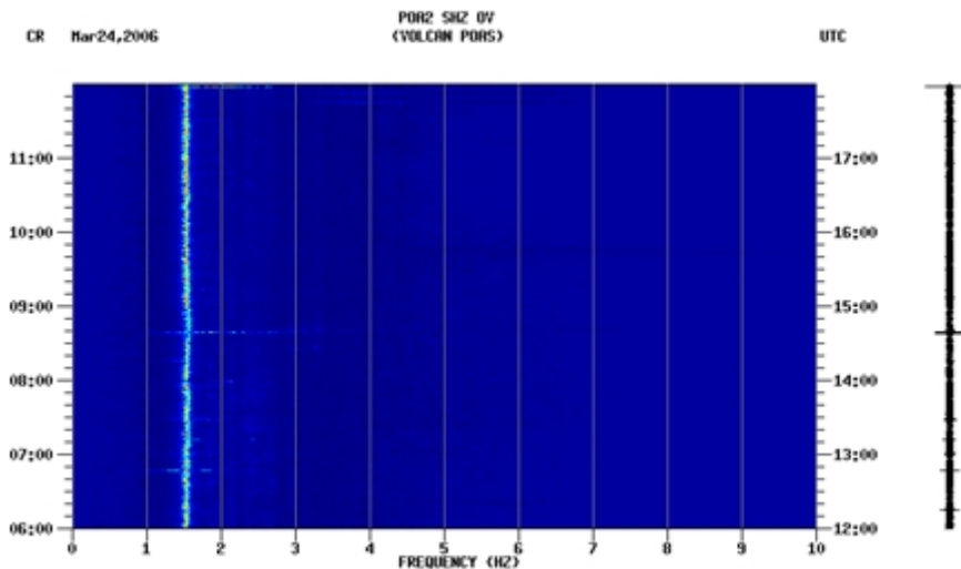
Figura 10: Señal sísmica y espectrograma correspondiente a la primera erupción freática ocurrida a las 17:57 hrs GMT del 24 de marzo de 2006 (medio día hora local). La señal sísmica en el espectrograma se encuentra ubicada en la parte superior del espectrograma con una frecuencia dominante de 2.8 Hz. La frecuencia dominante en el resto del espectrograma corresponde a tremor monocromático armónico.
