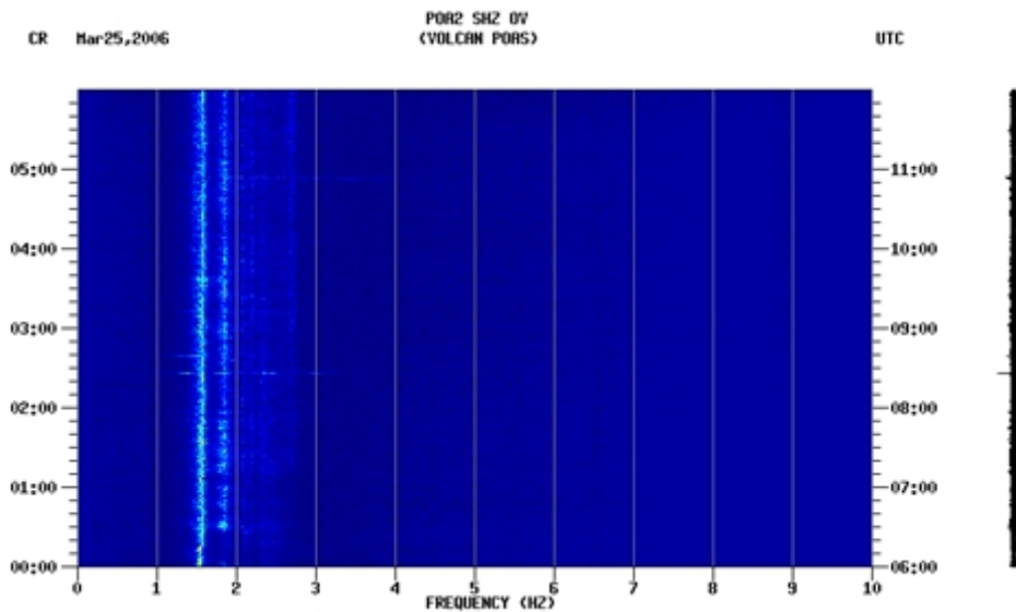
Figura 12: Espectrograma del tremor policromático con frecuencias dominantes de 1.5 Hz y 1.8 Hz. Este tremor comenzó a ser registrado el 25 de marzo de 2006 a las 06:26 hrs GMT.
