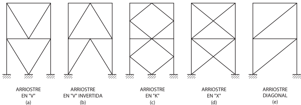
Fig. 10.1. Marcos arriostrados concéntricamente, ref. 7.
