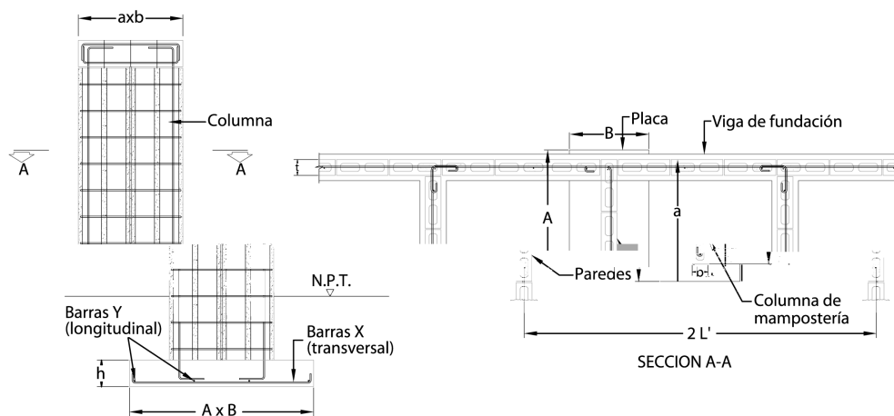
Fig. 17.27. Detalle de columnas de mampostería con refuerzo integral.
