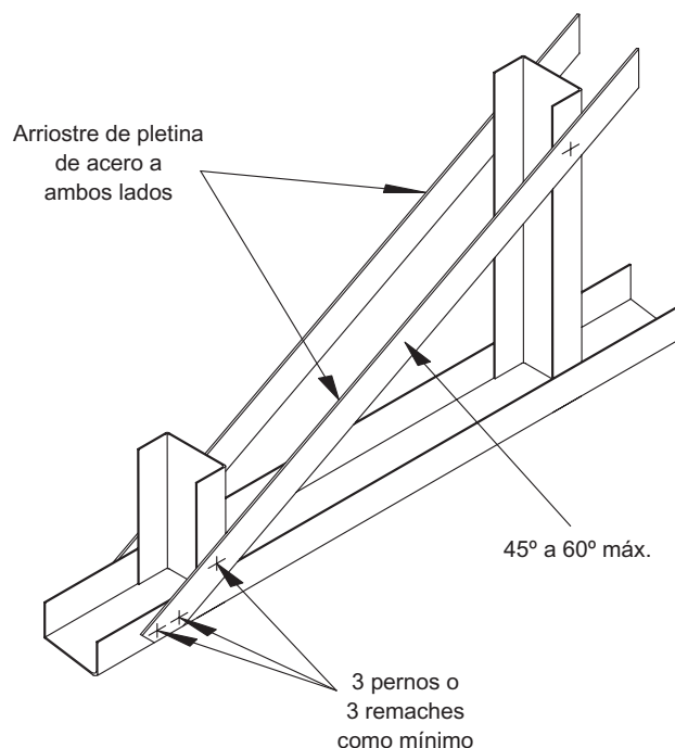
Fig. 17.19. Arrioste de paredes a doble forro.
