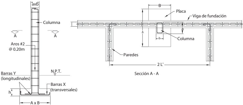
Fig. 17.26. Detalle de columna de concreto reforzado para rigidizar paredes.
