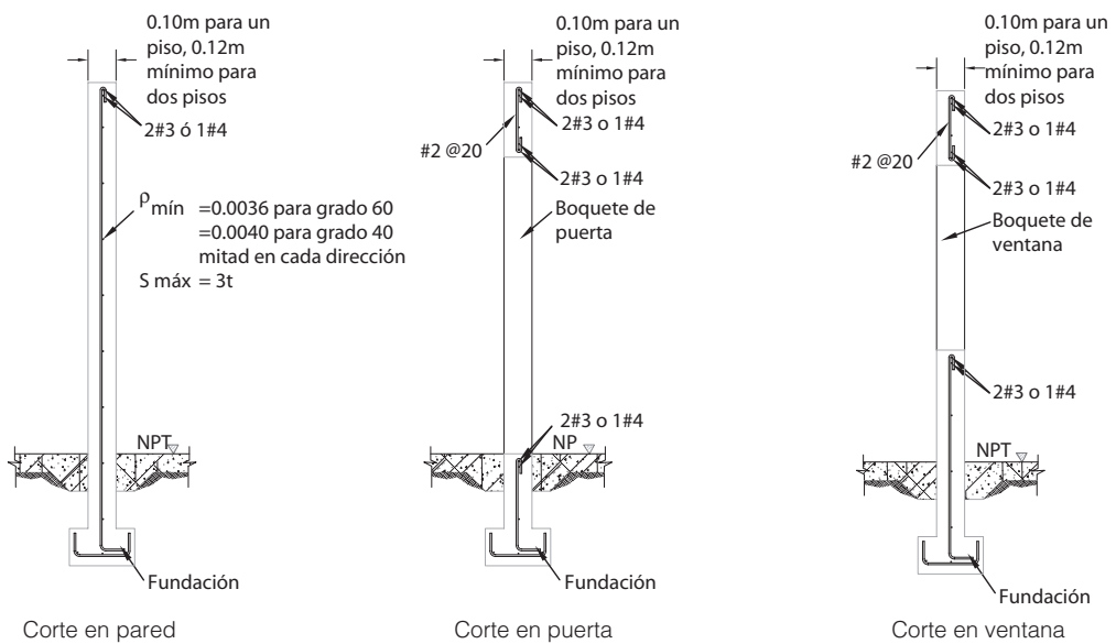
Fig. 17.14. Cortes en paredes de concreto reforzado.
