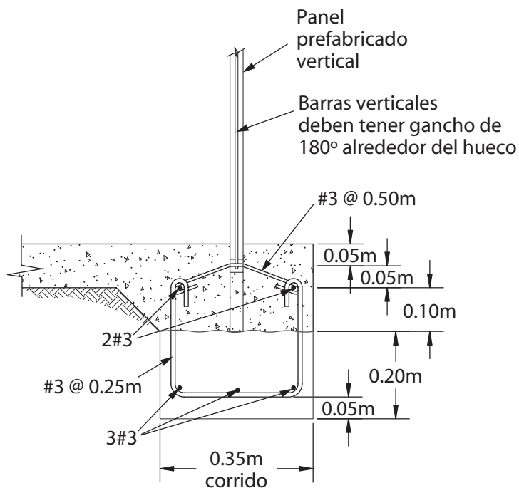
Fig. 17.3. Fundación para baldosas verticales
